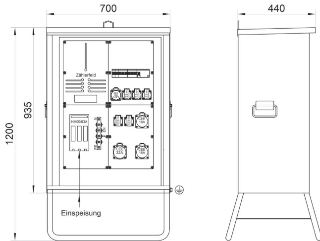
STVZ 63 I max : 63A
