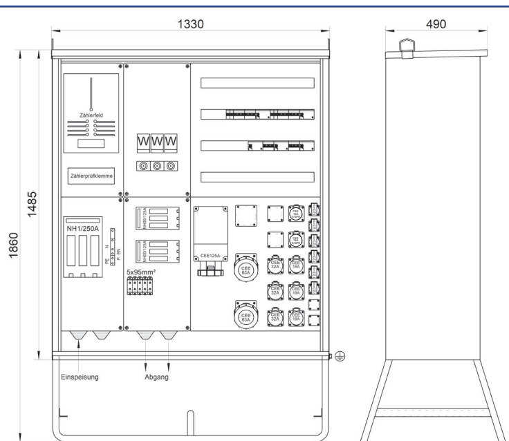
STVZW 250 I max : 250A
