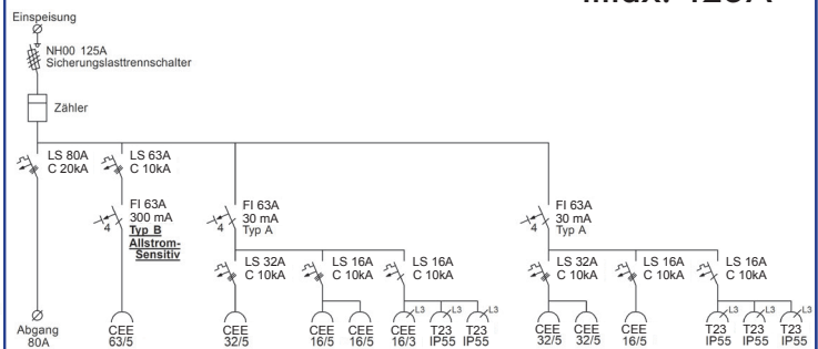
STVZ 125 I max : 125A
