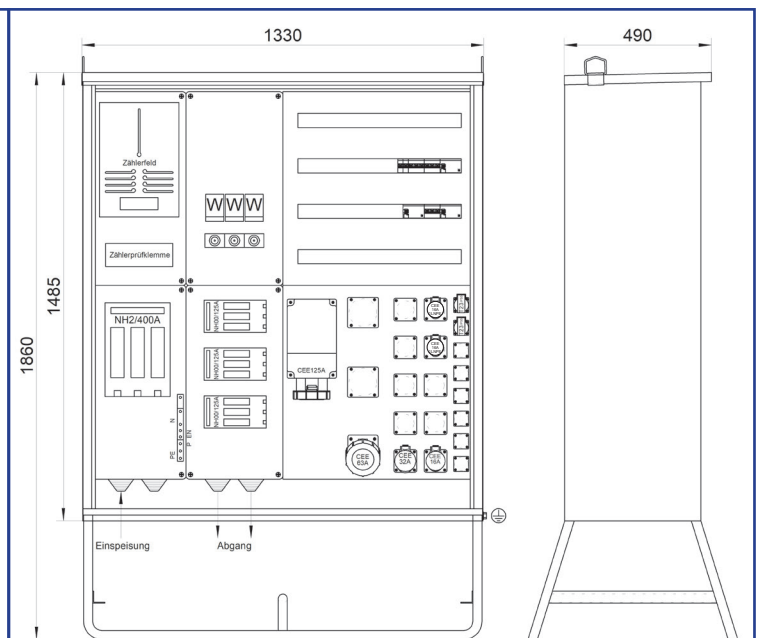
STVZW 400 I max : 400A
