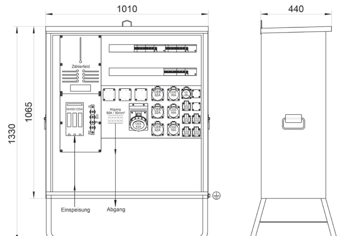
STVZ 125 I max : 125A
