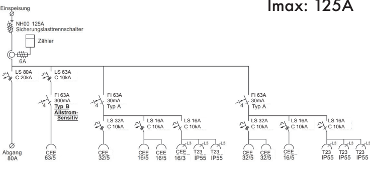
STVZW 125 I max : 125A
