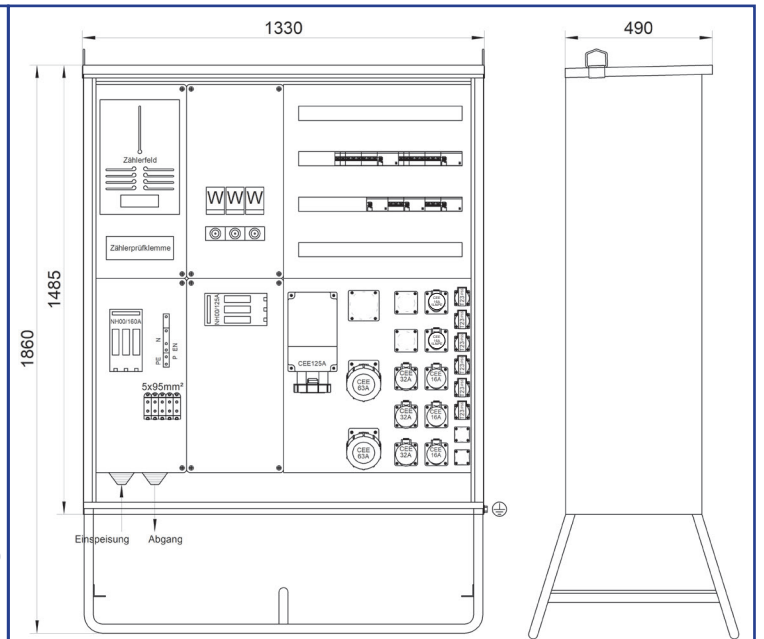
STVZW 160 I max : 160A
